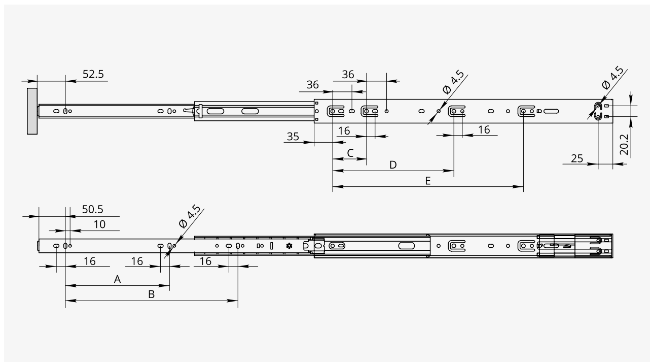
Установочные размеры
