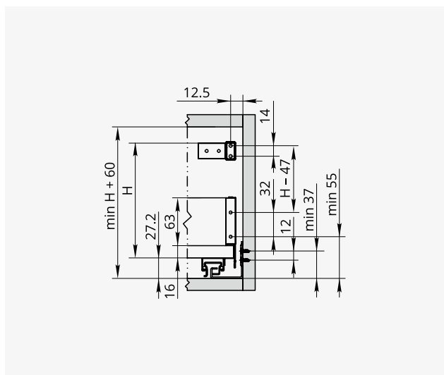
Схема присадки ящика H=131
