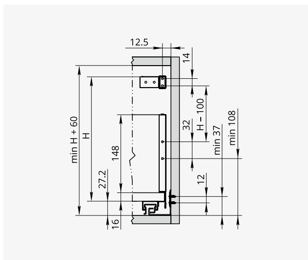
Схема присадки ящика H=178
