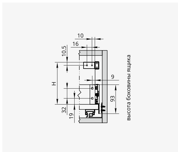
Схема присадки задней панели ящика H=131
