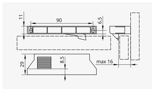
Размеры ручки-поводка 8.5 – 16 мм
