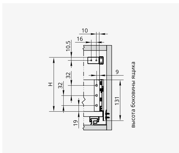
Схема присадки задней панели ящика H=178
