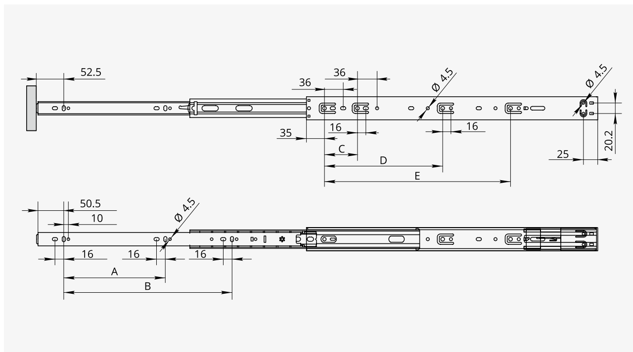
Установочные размеры
