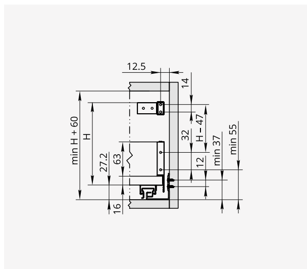
Схема присадки ящика H = 131
