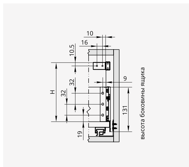
Схема присадки задней панели ящика H = 178
