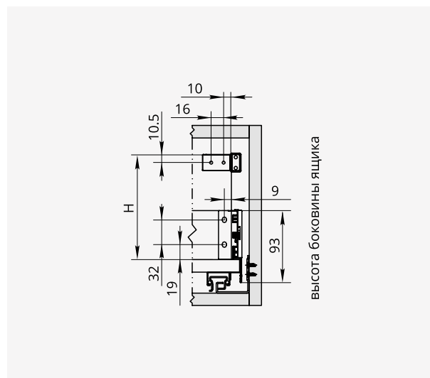
Схема присадки задней панели ящика H = 131
