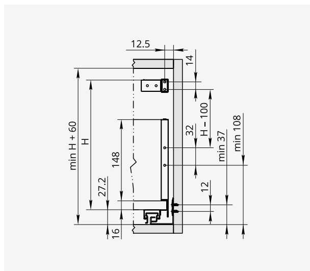
Схема присадки ящика H = 178
