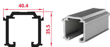
Верхняя направляющая
