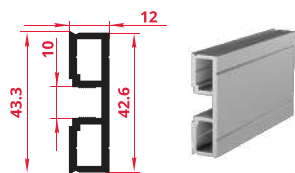
Вертикальный профиль
