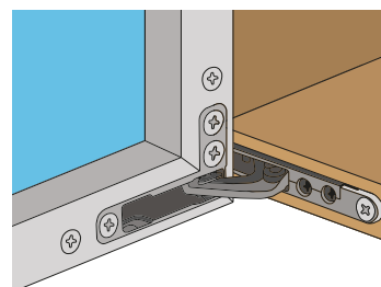
Установка нижней петли
