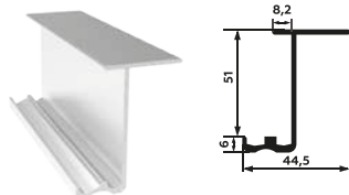
ВЕРХНЯЯ НАПРАВЛЯЮЩАЯ
