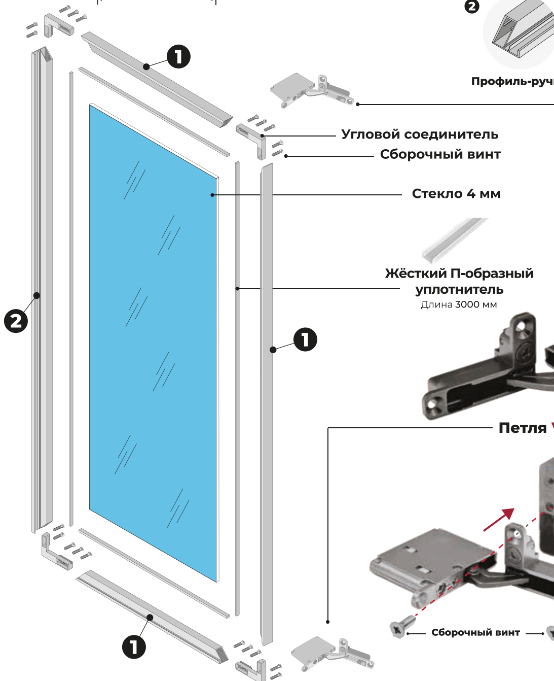
Рамочный профиль TORO
