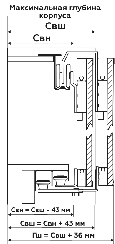
Максимальная глубина шкафа для рамочной системы
