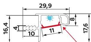
Крышка-рассеиватель
