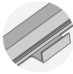
Профиль-ручка MANTO / PICO
