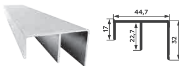
НИЖНЯЯ НАПРАВЛЯЮЩАЯ
