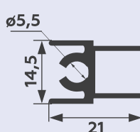
ВЕРХНИЙ ГОРИЗОНТАЛЬНЫЙ ПРОФИЛЬ
