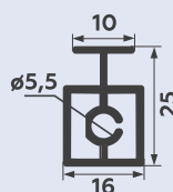
ДВУСТОРОННИЙ ПРОФИЛЬ ELEPHANT
