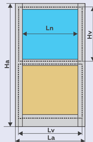
РАЗМЕРЫ ДВЕРИ
